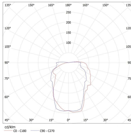
KANLUX S.A. (kat 08050) SANGA DL-100 / Krzywa rozsyłu światła (biegunowo)
